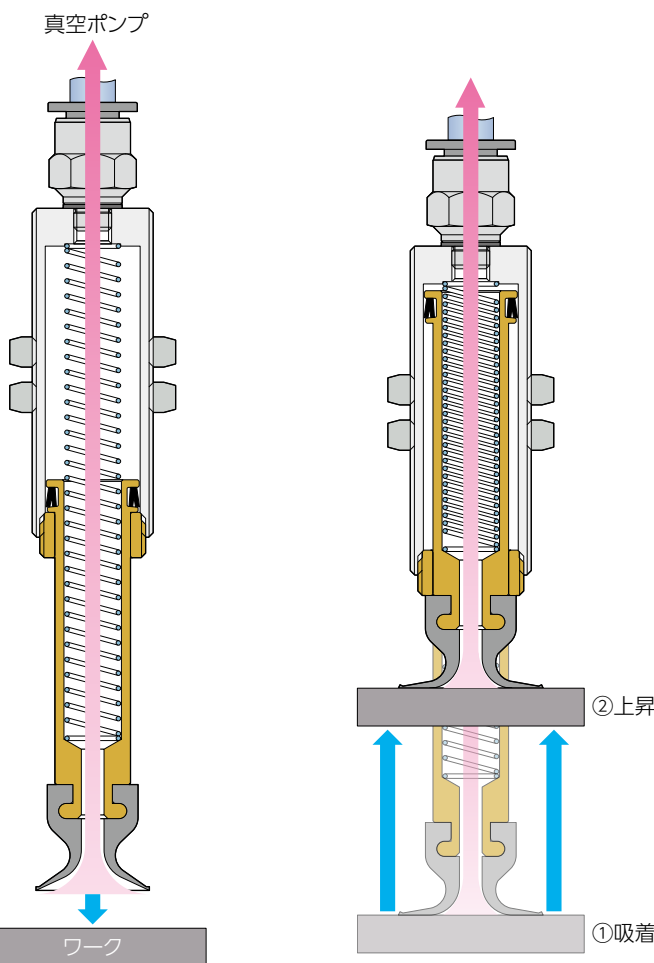
形式例 VSP10-30LN6J ↳ 真空ポンプ仕様
